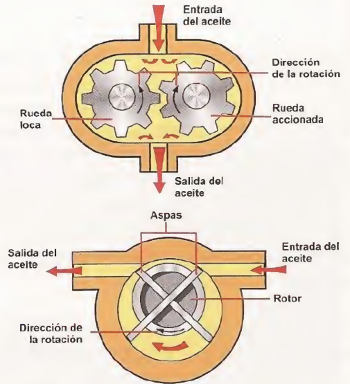
Bomba de aceite tipo engranaje piñón - piñón
